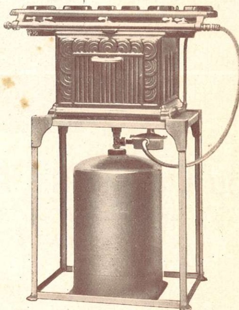
Type N° 4 B. pour réchauds four
