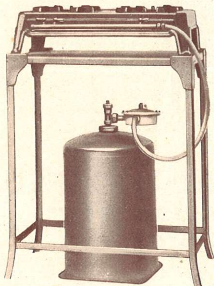
Type N° 2 B. pour réchauds plats 2 feux
